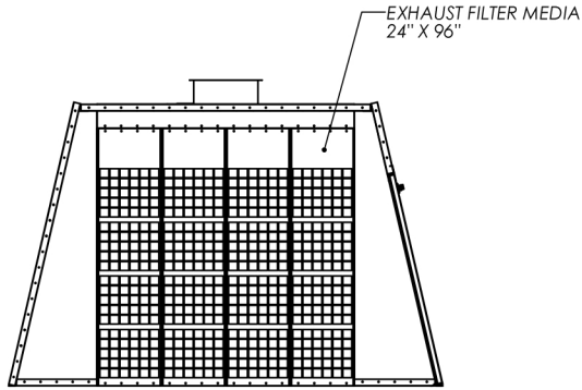
SECTION A-A SCALE 1 : 35
